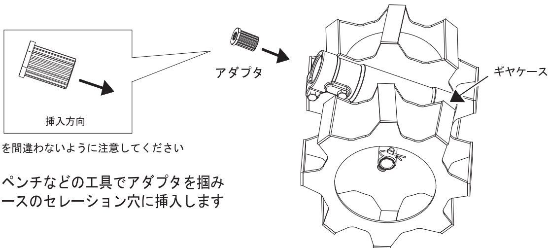
ギヤケースのセレーション穴
